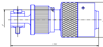
Розетка кабельная с прямым кожухом
