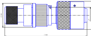
Розетка кабельная с обложкой под термоусаживающиеся трубки
